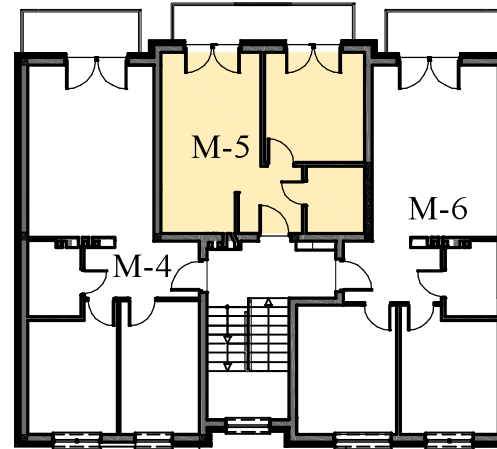
RZUT KONDYGNACJI - I PIĘTRO
