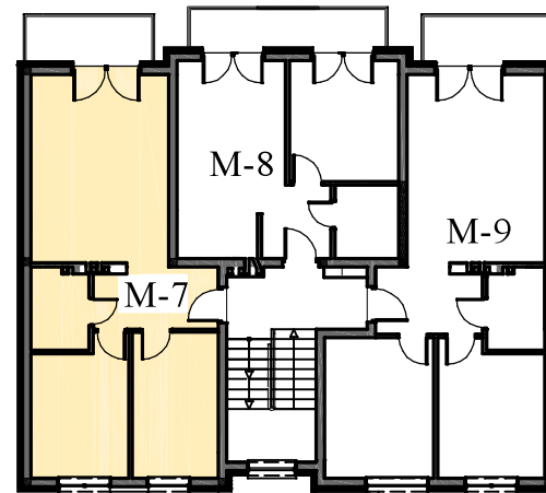
RZUT KONDYGNACJI - II PIĘTRO
