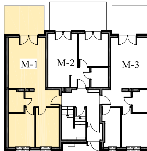
RZUT KONDYGNACJI - PARTER
