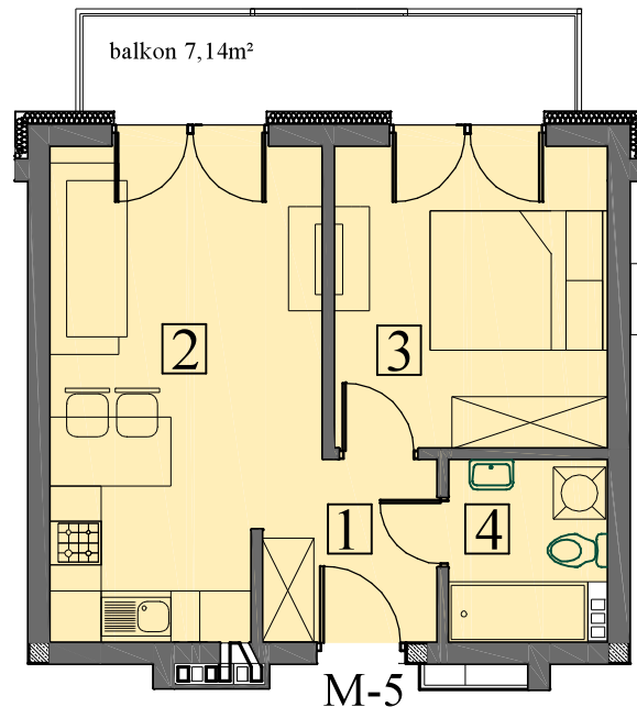
RZUT MIESZKANIA M5
