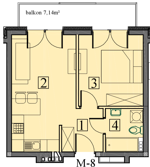
RZUT MIESZKANIA M8
